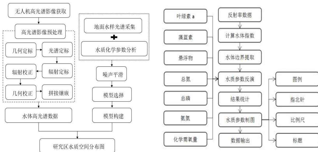
无人机高光谱水环境监测技术路线图
