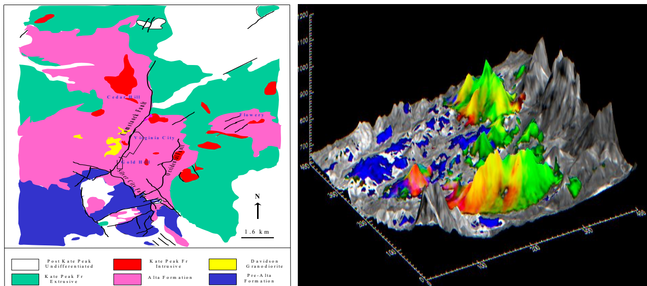
矿物填图与 DTM 制图
